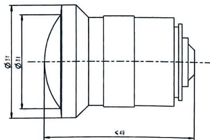
图 1 鱼眼镜头尺寸示意图
